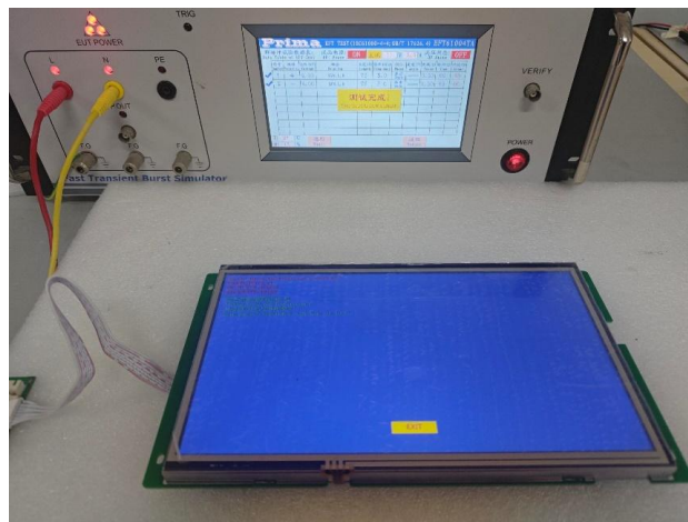
图 4-3 EFT 测试
