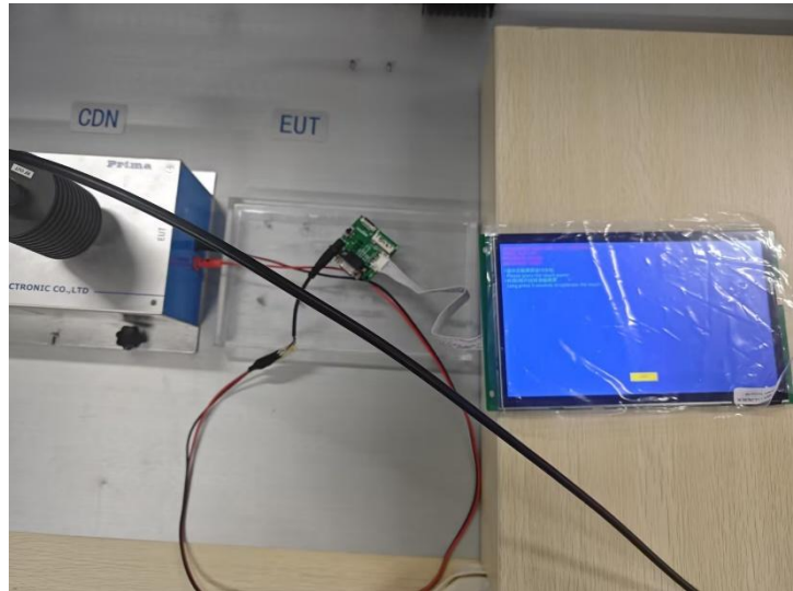
图 4-4 CS 测试图
