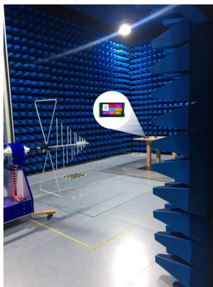
图 4-5 RE 测试图
